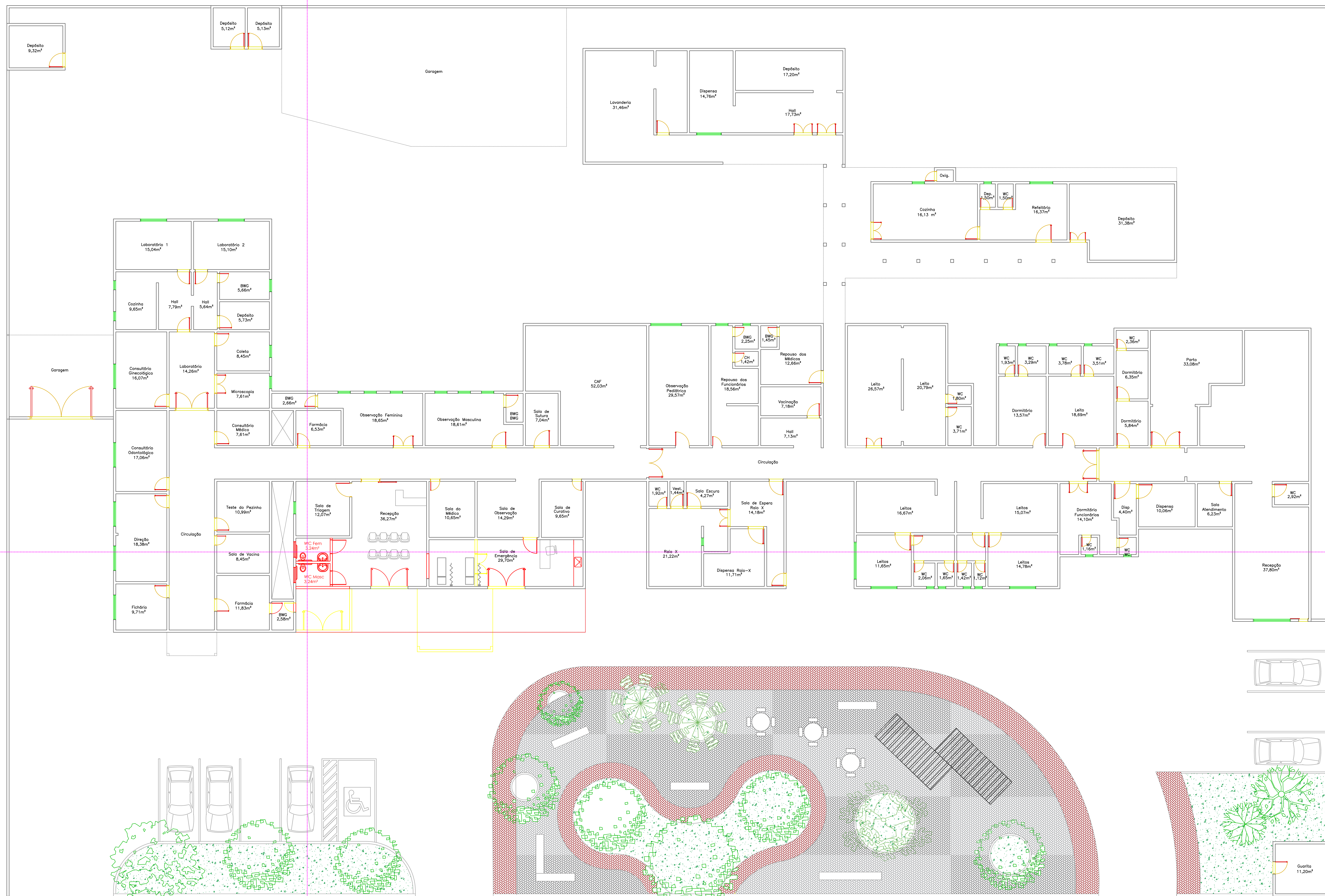
02 PLANTA DE REFORMA ESCALA 1/150
